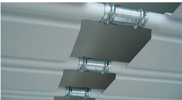
Speziell entwickelte Sunline Schiebemuffen ermöglichen das Verpressen der Einzelplatten zu langen Bändern
